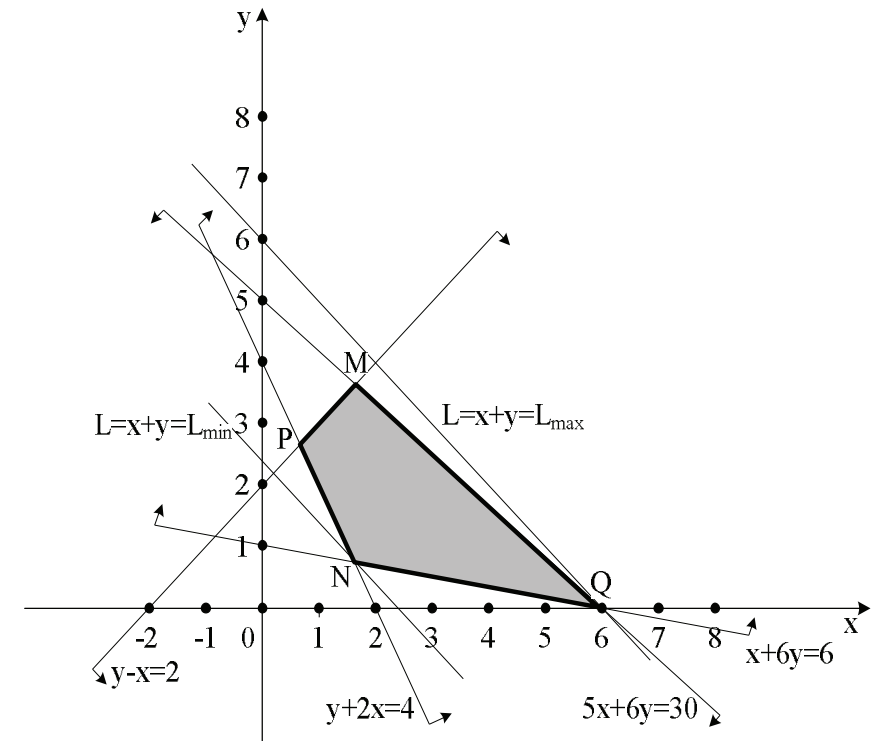
Рис.3. К примеру 15. Геометрическая интерпретация задачи линейного программирования
